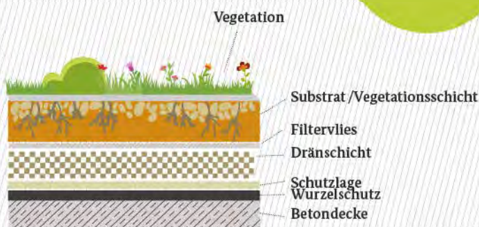
Aufbau eines Gründaches als Kaldach
